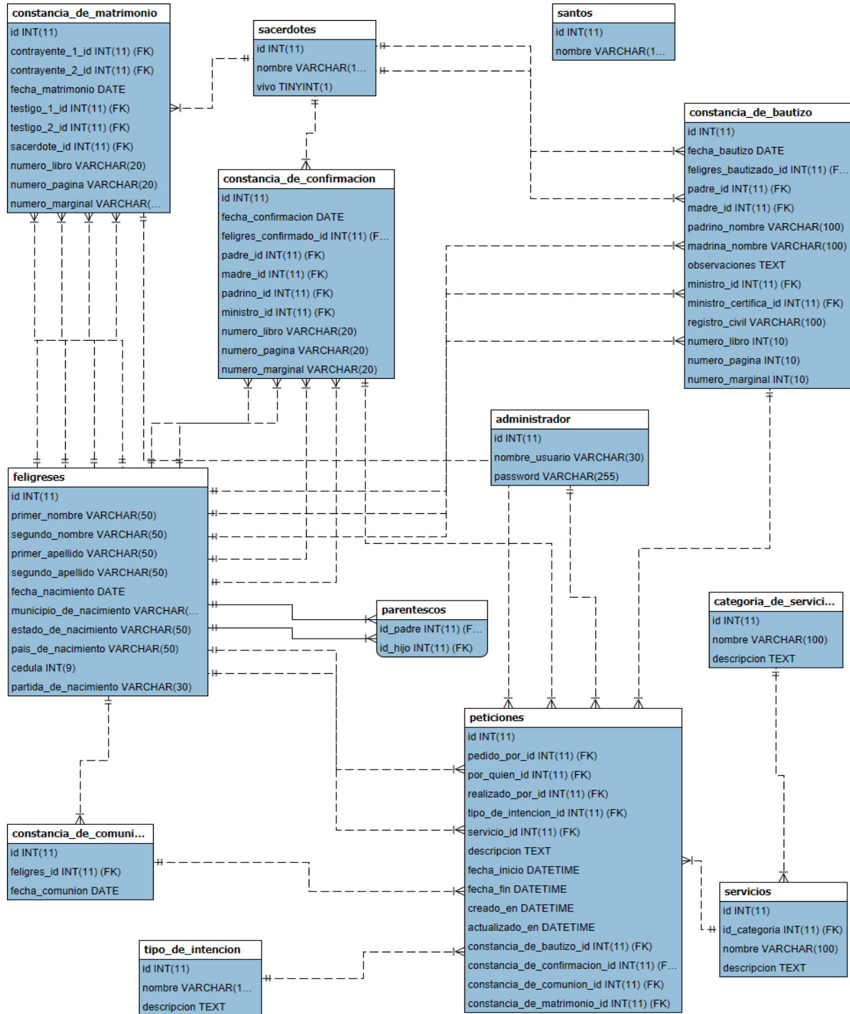
Grafico 1. Diagrama de Datos del sistema.
